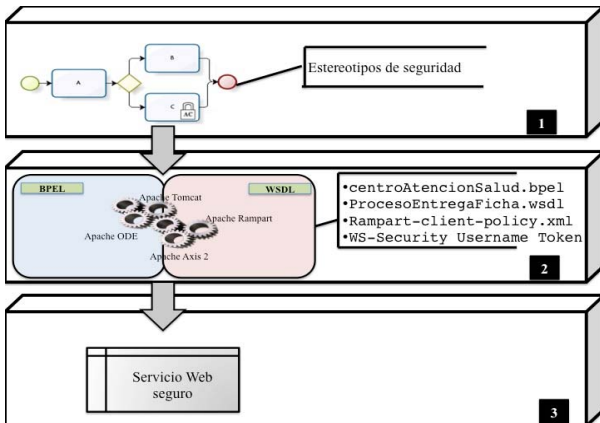
Figura 4. Aspectos técnicos para obtener servicios Web Seguro desde un SBP
