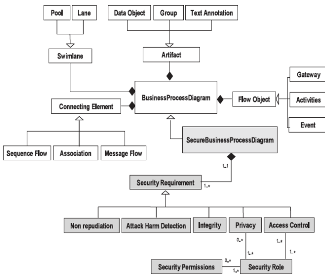
Figura 1. Metamodelo BPMN extendido con requisitos de seguridad [16].
