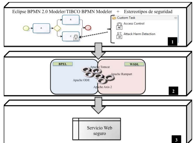
Figura 2. Propuesta de integración de la seguridad en BPEL desde un BPMN seguro.
